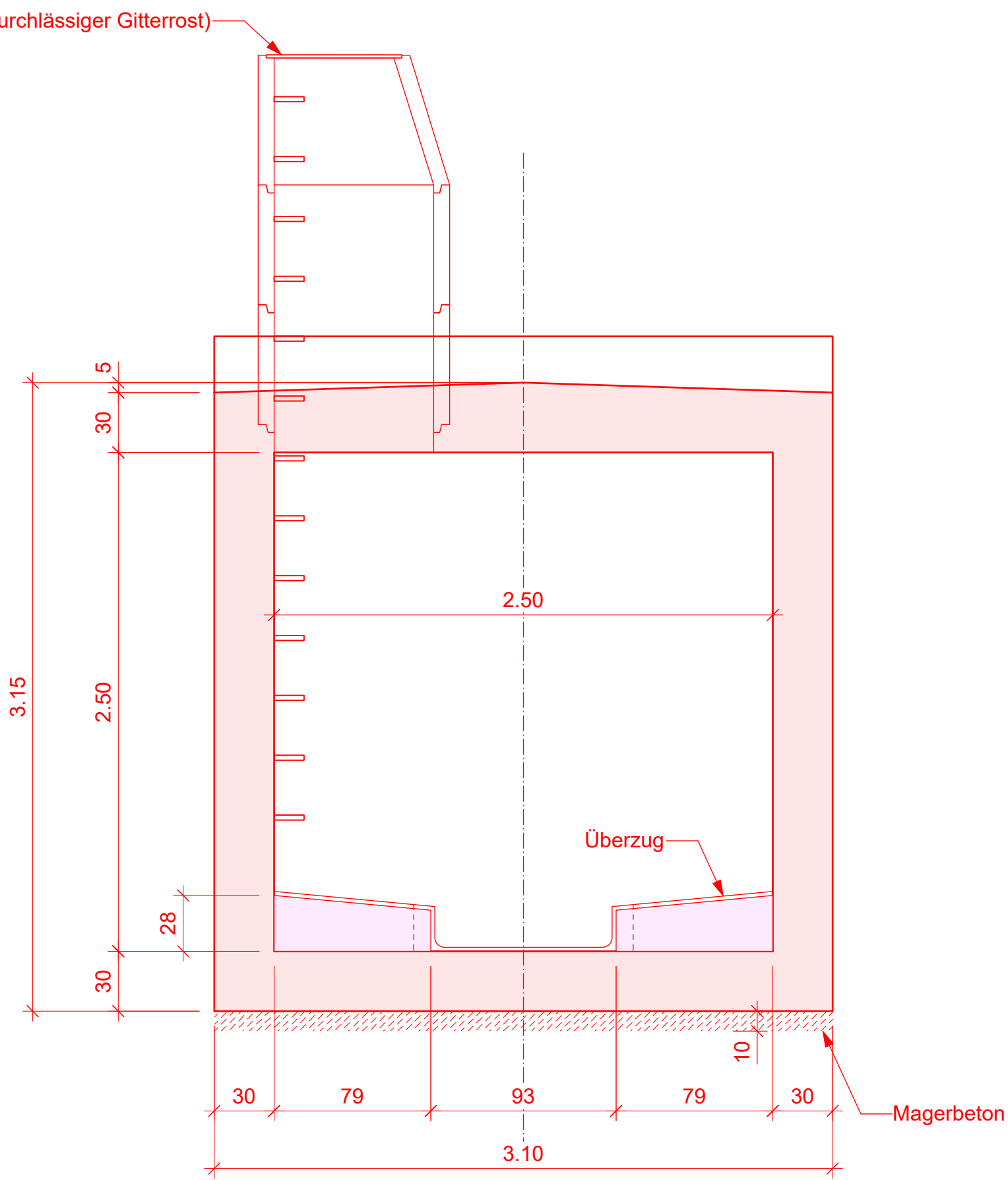
Schnitt C - C (1:25)
