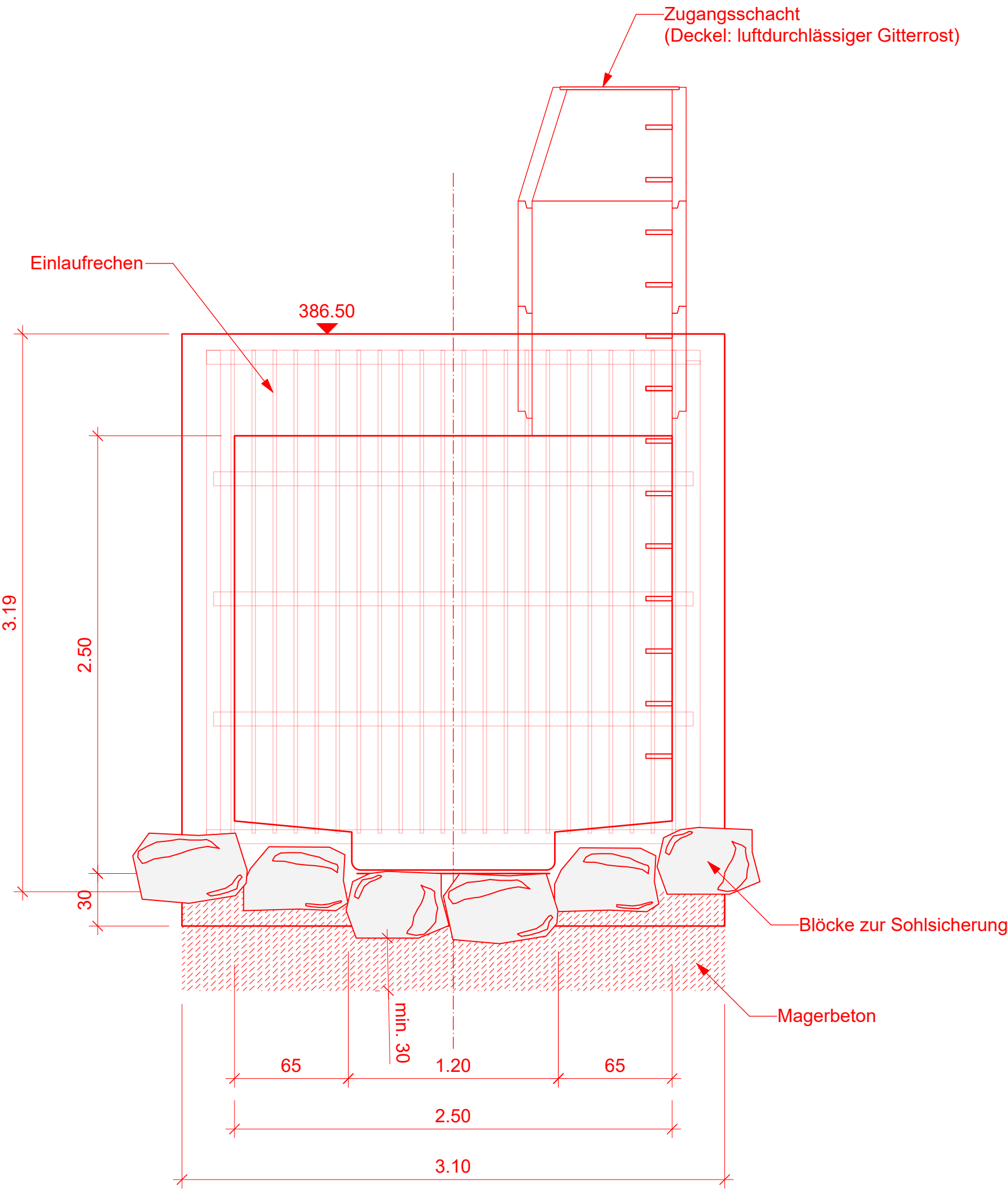
Schnitt D - D (1:25)
