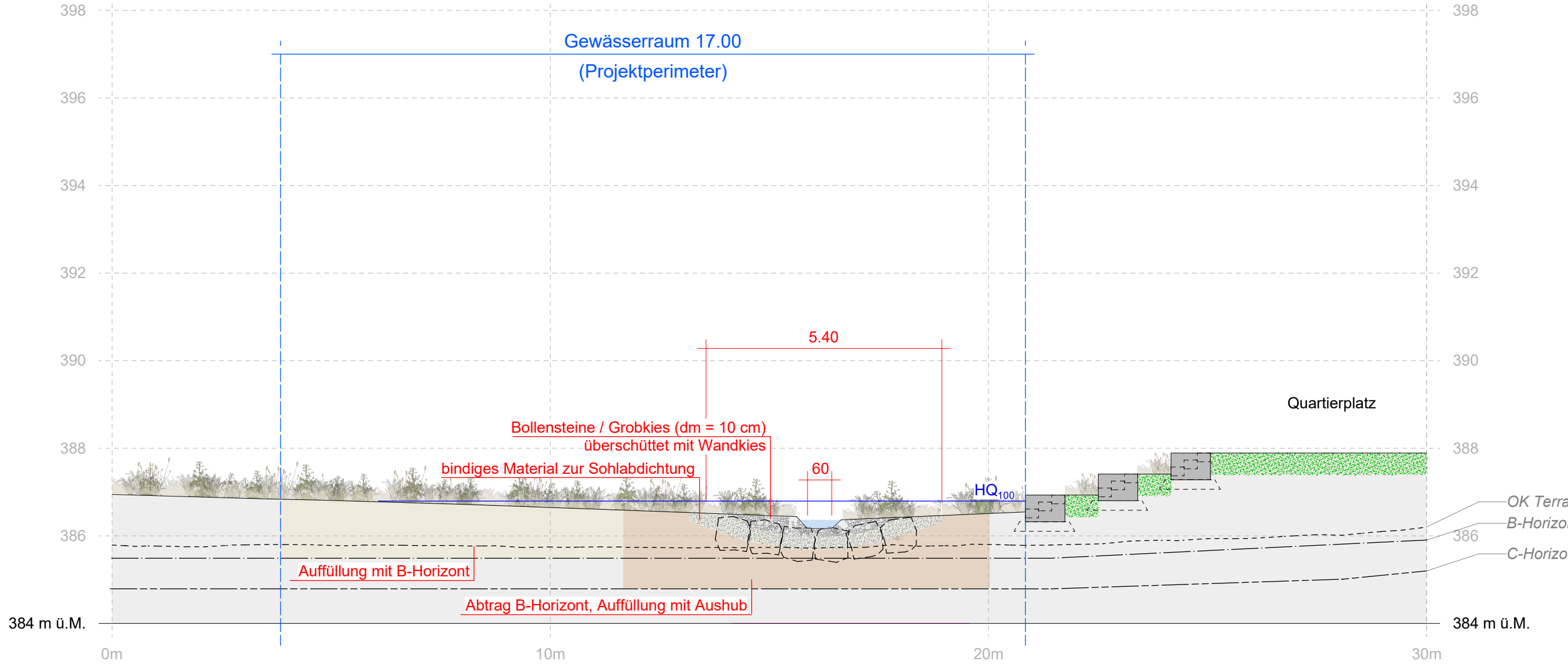
Querprofil 4, Quartierplatz (Metrierung 520m)
