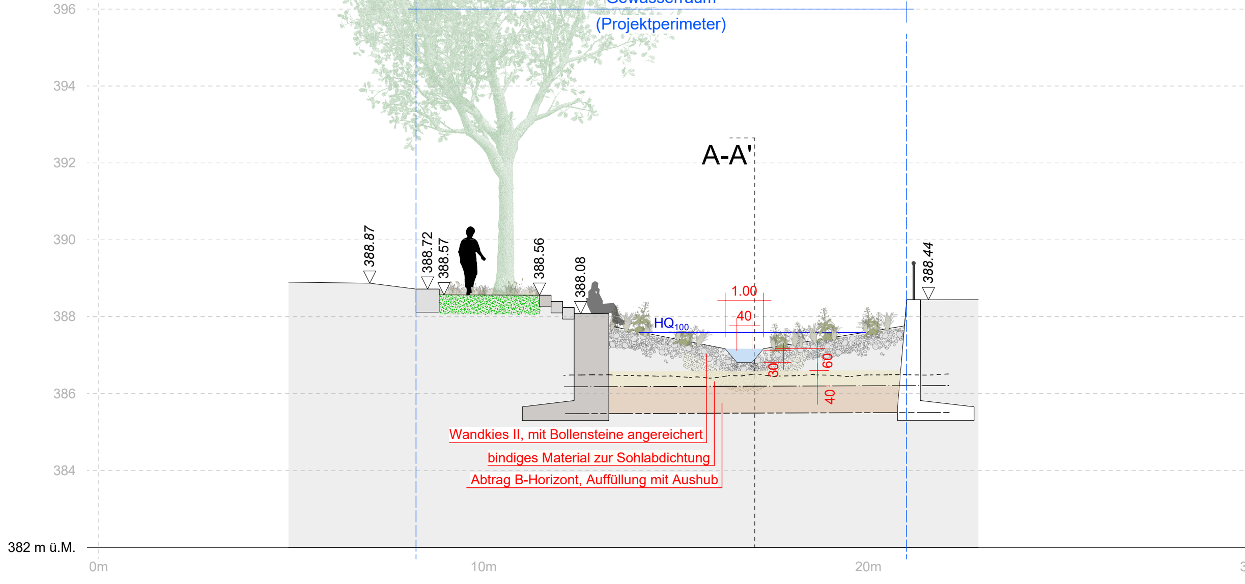
Querprofil 5, Maienplatz (Metrierung 578.7m)
