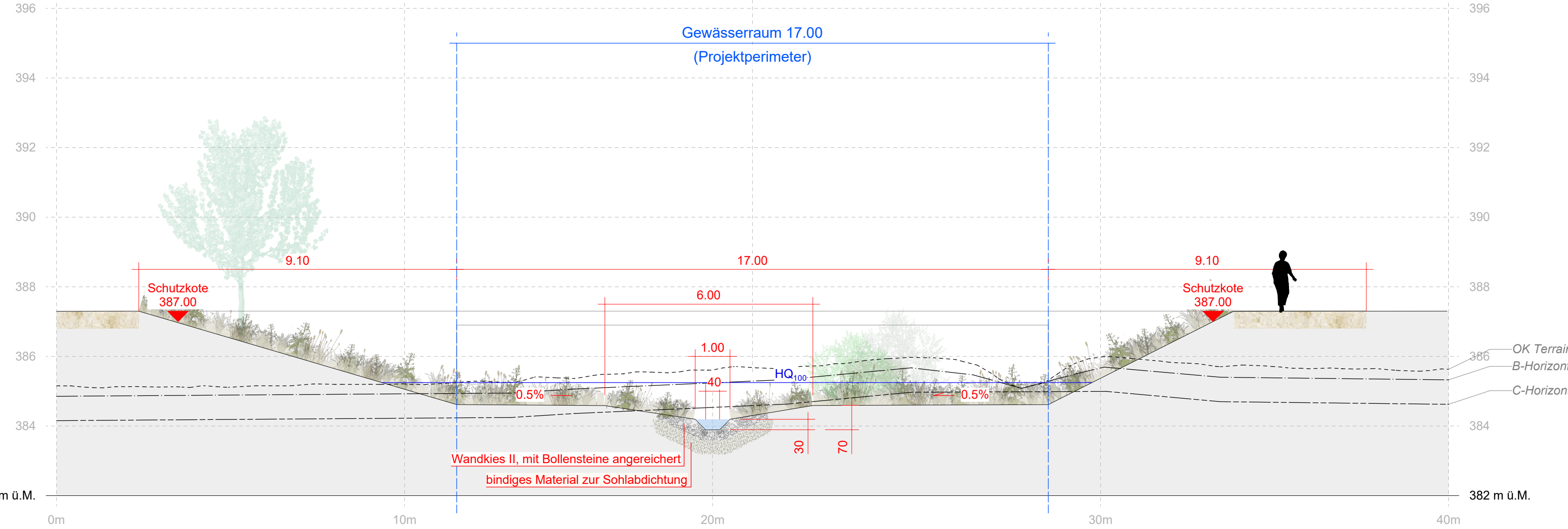
Querprofil 1, Park (Metrierung 125m)
